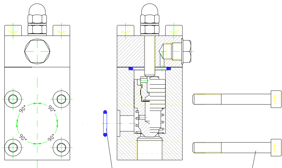
Viti di fissaggio Fixing screw M8 x 60 8.8
