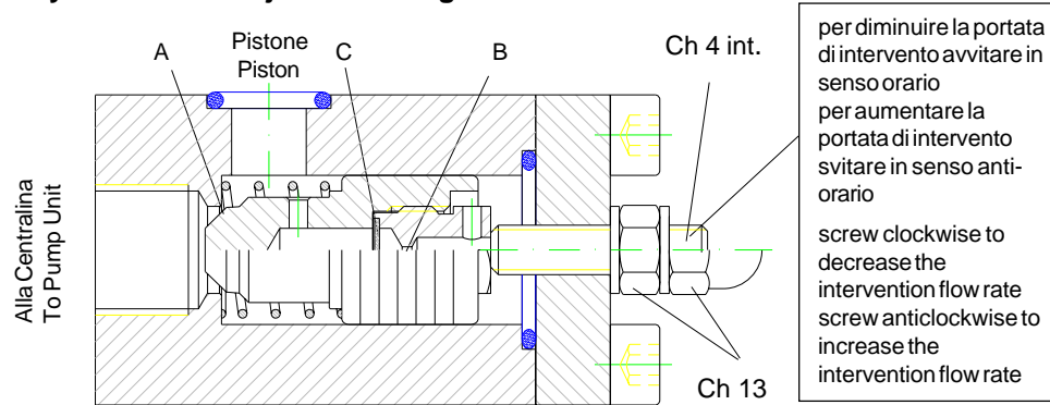
A - Sezione di regolazione velocita' di intervento - Operating flow adjusting section B - Sezione di controllo della velocita' di chiusura - Section of control of closing speed C - Filtro - Filter
