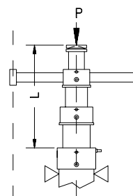
Pistone con una guida es. 58/3 g 1
