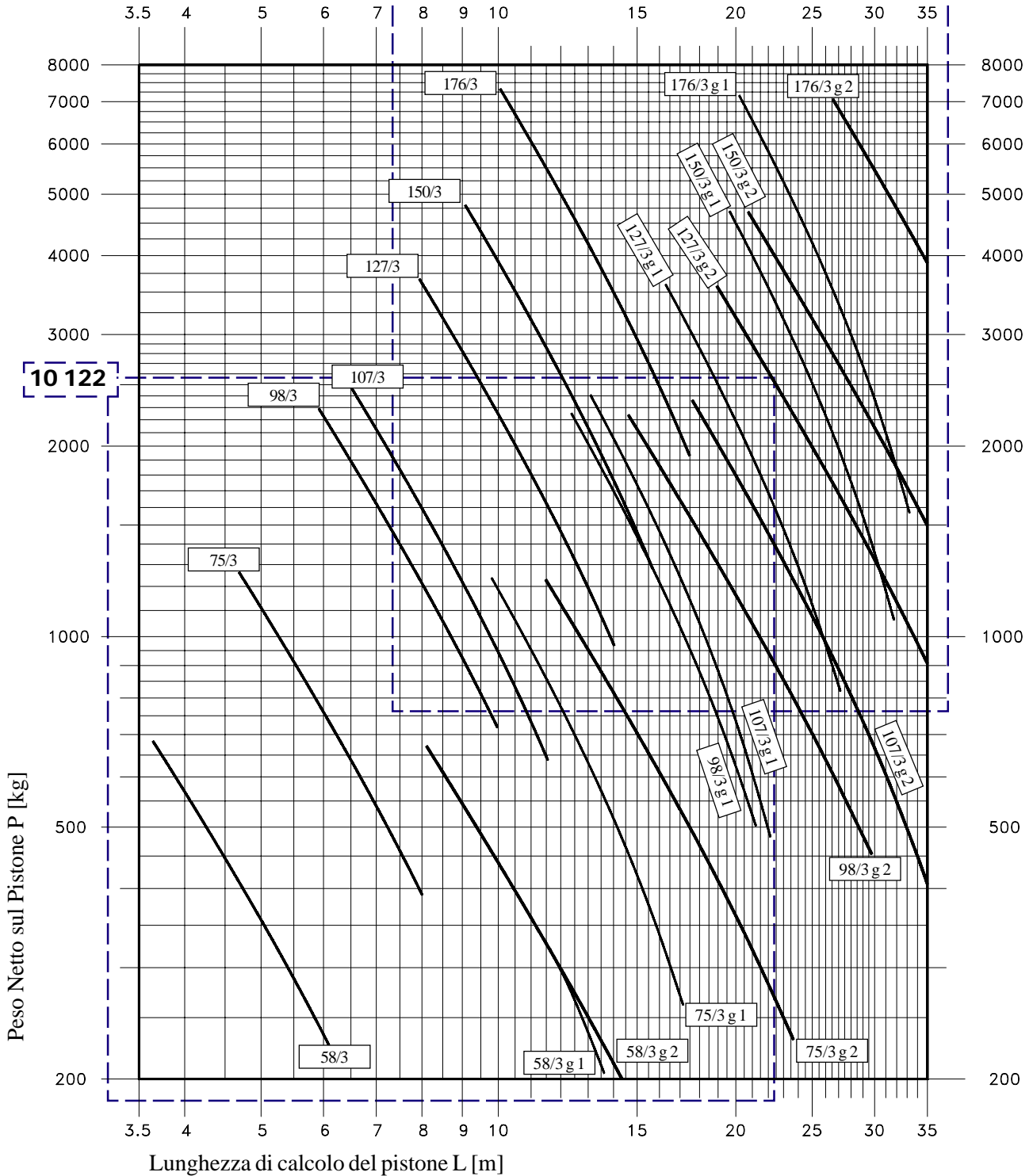
Pistone senza guide es. 58/3
