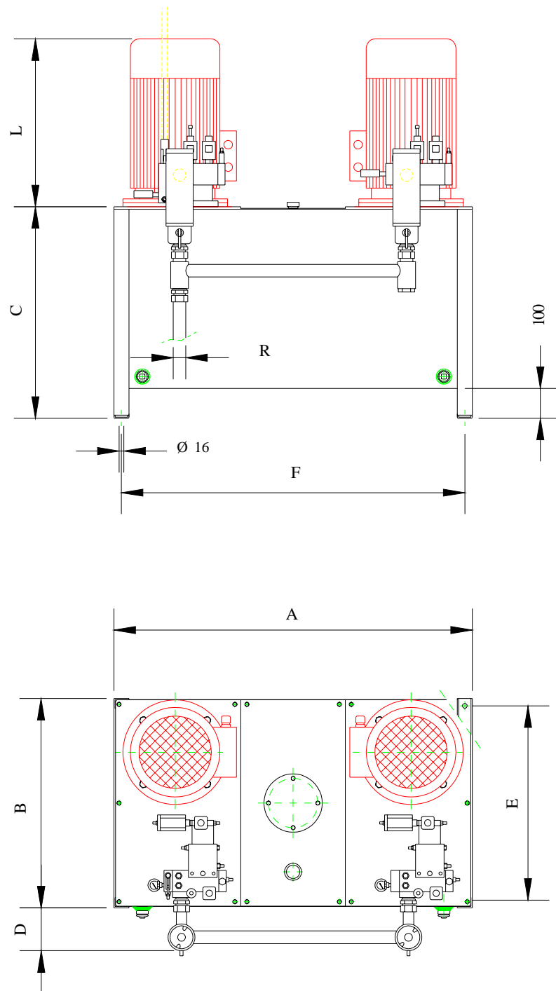
DOPPIO GRUPPO MOTORE-POMPA (2MP)
